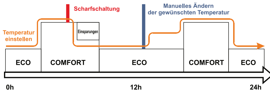
Abb. 6: Entwicklung der Temperaturen für einzelne Systemaktionen
